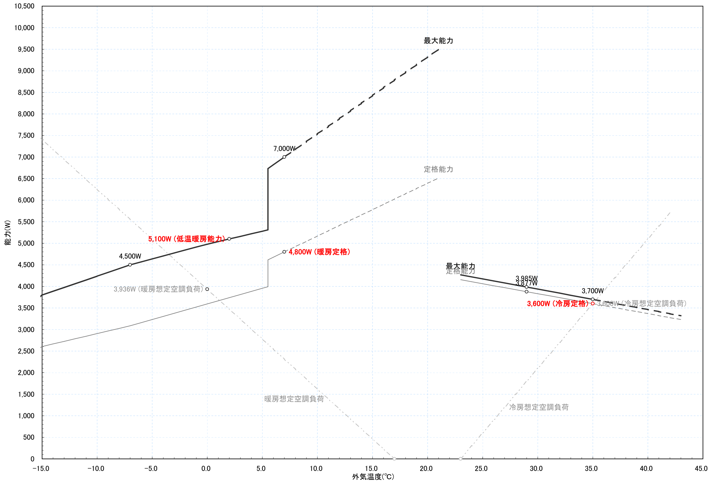
RAF-D36C 冷暖房能力特性図 [室温:冷房:27°C一定, 暖房:20°C一定]
