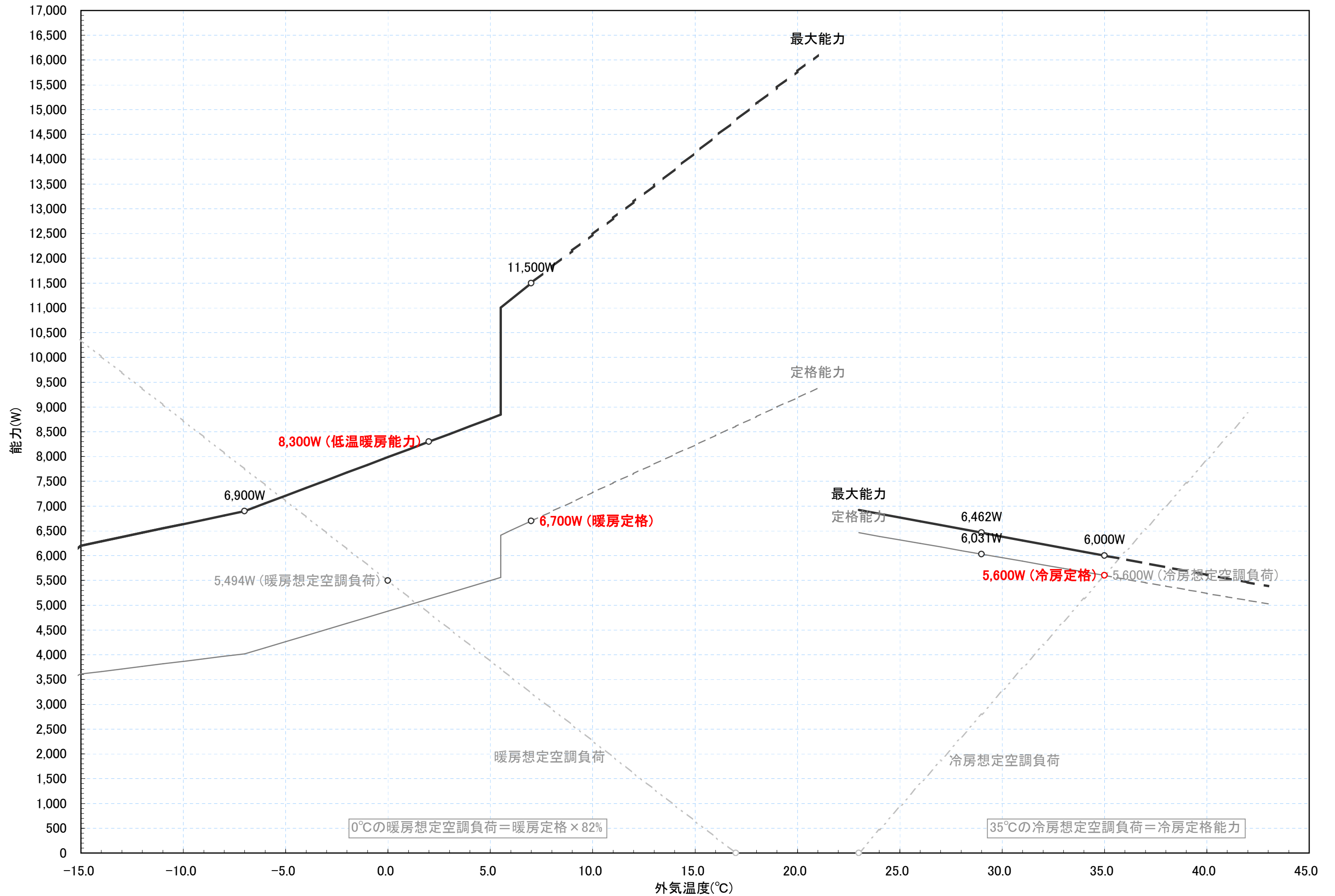
RAS-SK56A2 冷暖房能力特性図 [室温 冷房:27°C一定, 暖房:20°C一定]
