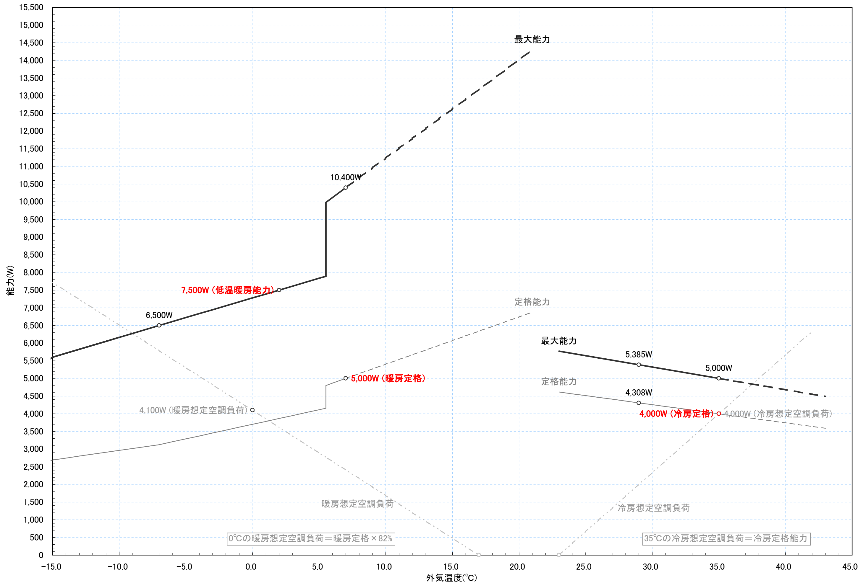
RAS-SK40A2 冷暖房能力特性図 [室温 冷房:27°C一定, 暖房:20°C一定]
