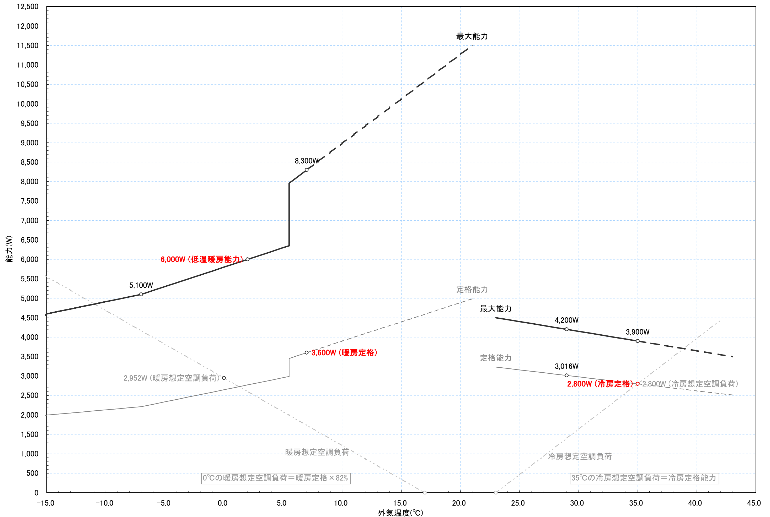
RAS-SK28A2 冷暖房能力特性図 [室温 冷房:27°C一定, 暖房:20°C一定]
