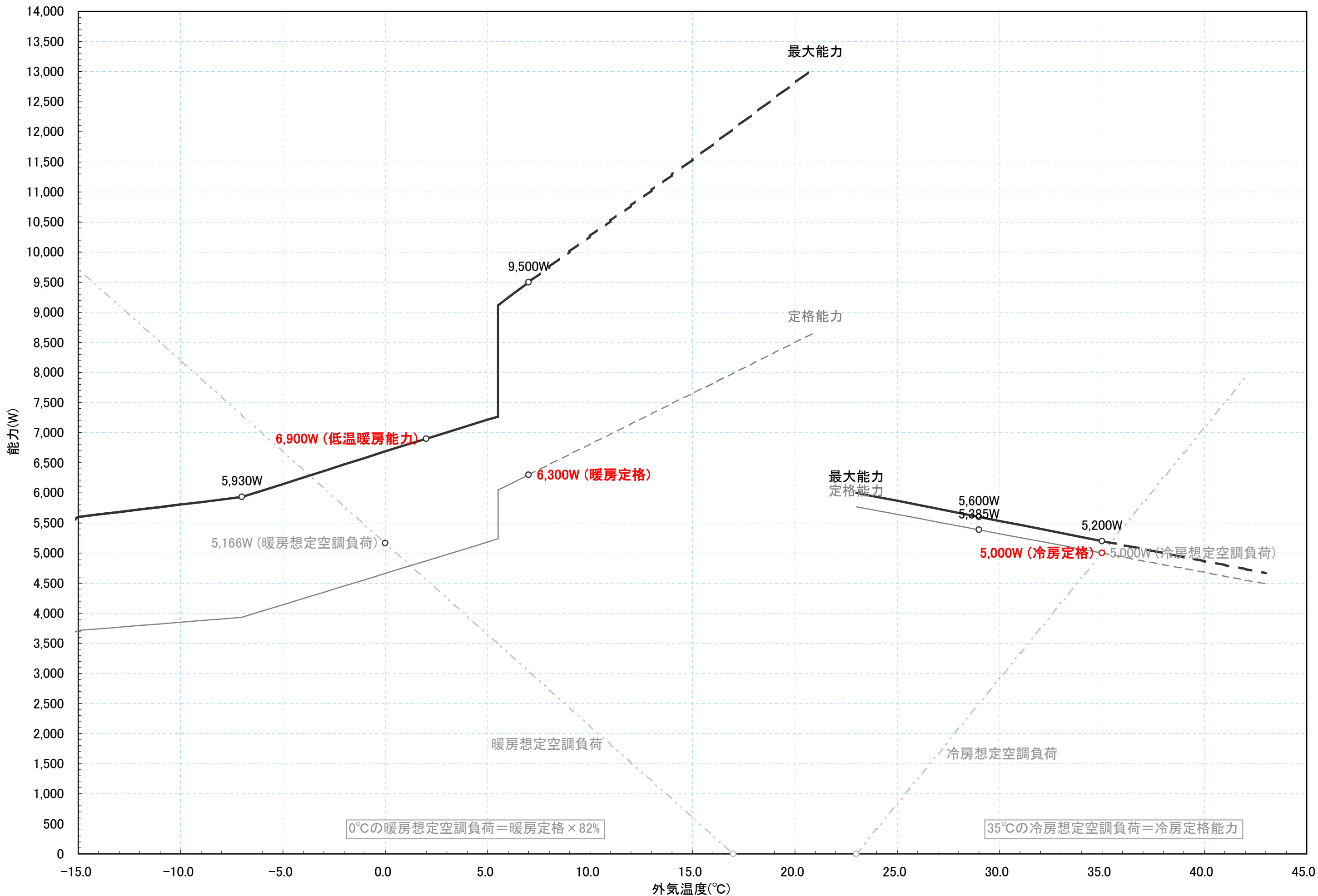
RAF-50A2 冷暖房能力特性図 [室温:冷房:27°C一定, 暖房:20°C一定]
