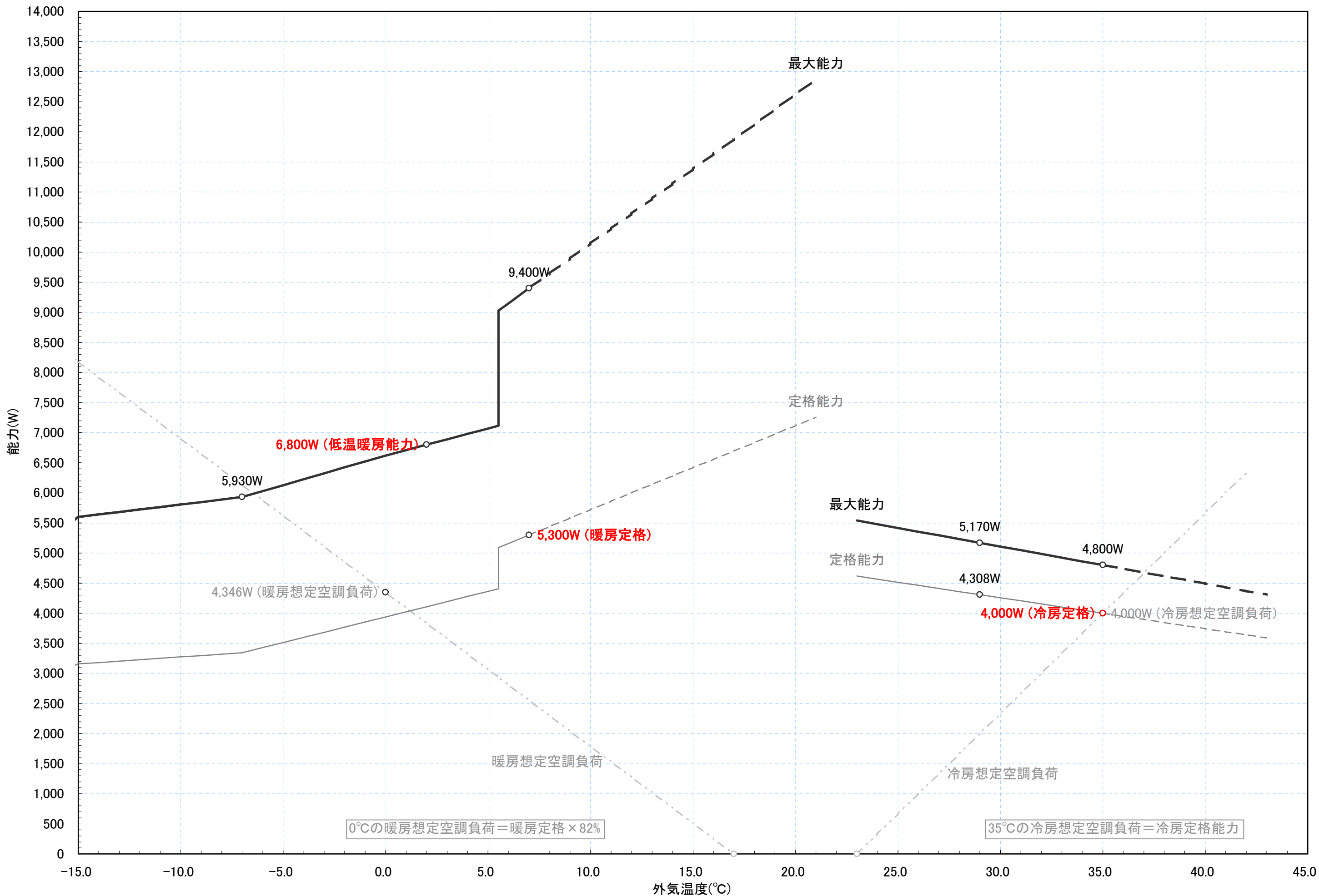
RAF-40A2 冷暖房能力特性図 [室温:冷房:27°C一定, 暖房:20°C一定]
