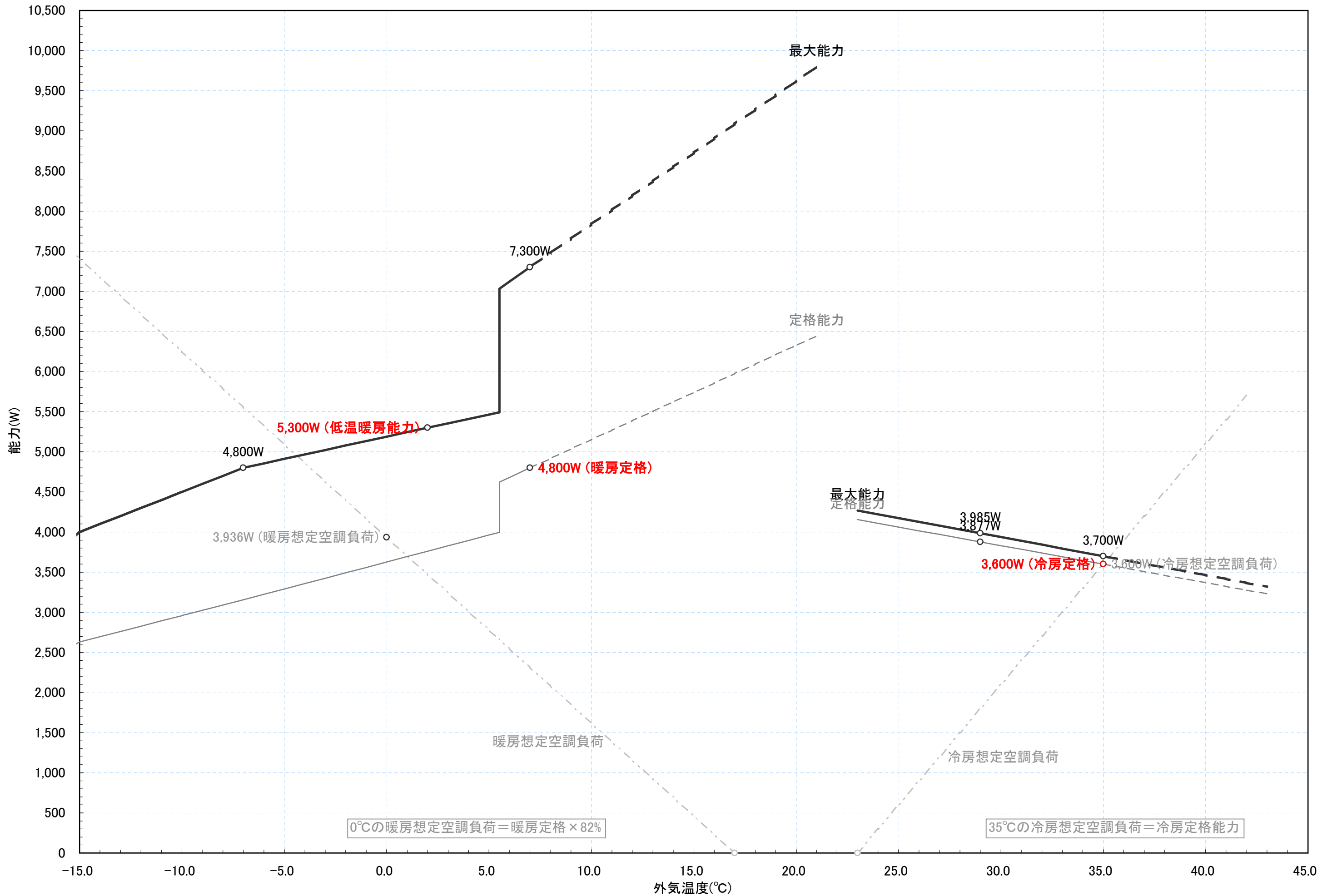
RAF-36A 冷暖房能力特性図 [室温:冷房:27°C一定, 暖房:20°C一定]
