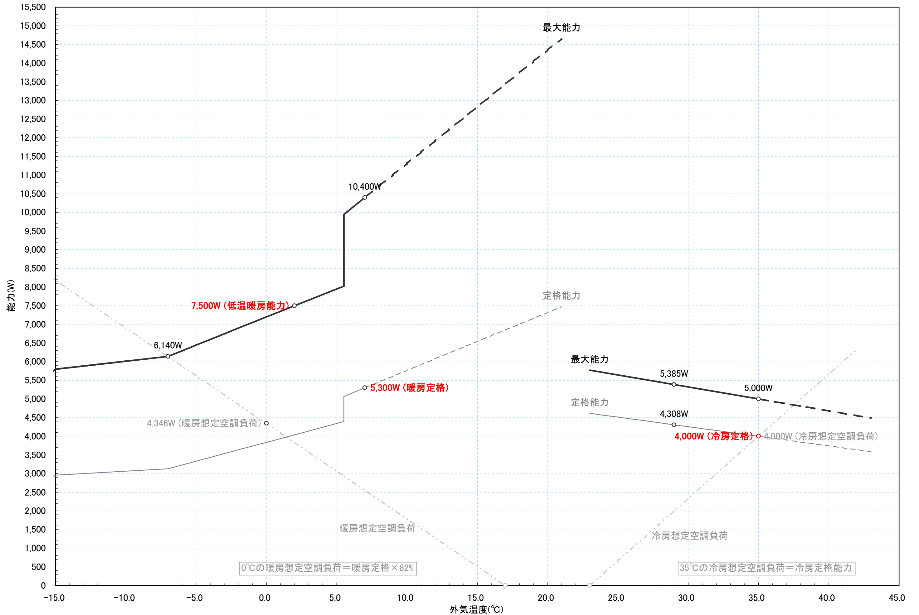
RAS-SD40Z2 冷暖房能力特性図 [室温 冷房:27°C一定, 暖房:20°C一定]
