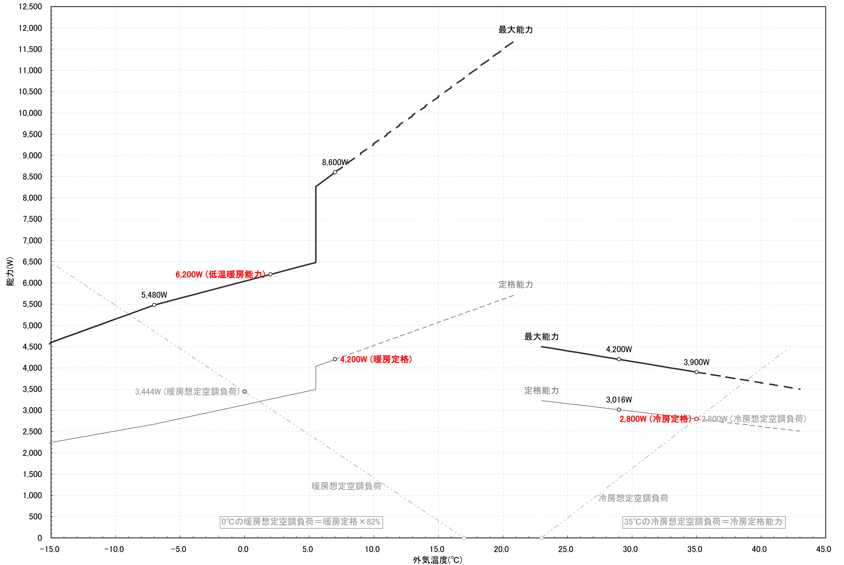
RAS-SD28Z2 冷暖房能力特性図 [室温 冷房:27°C一定, 暖房:20°C一定]
