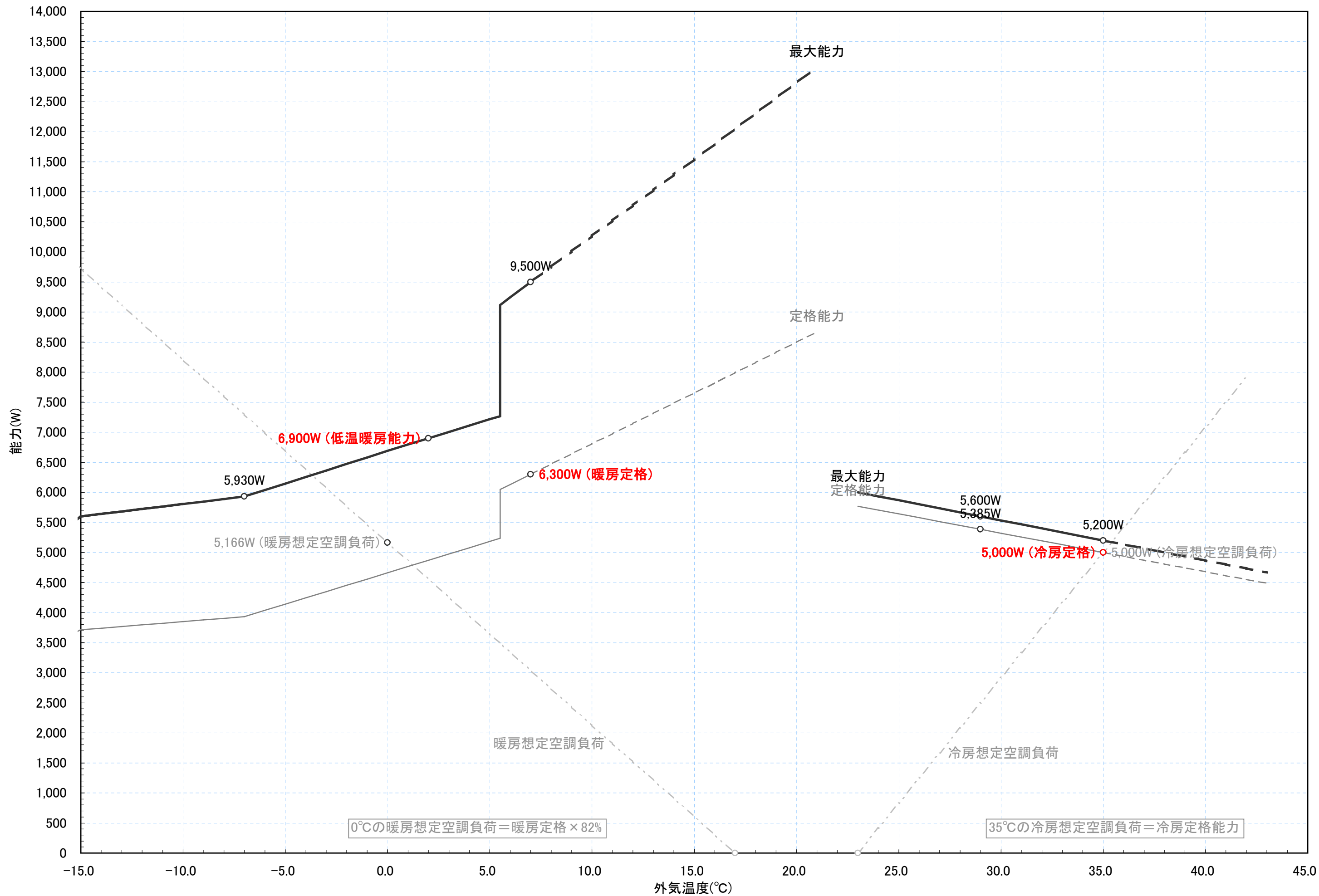
RAF-50Z2 冷暖房能力特性図 [室温 冷房:27°C一定, 暖房:20°C一定]
