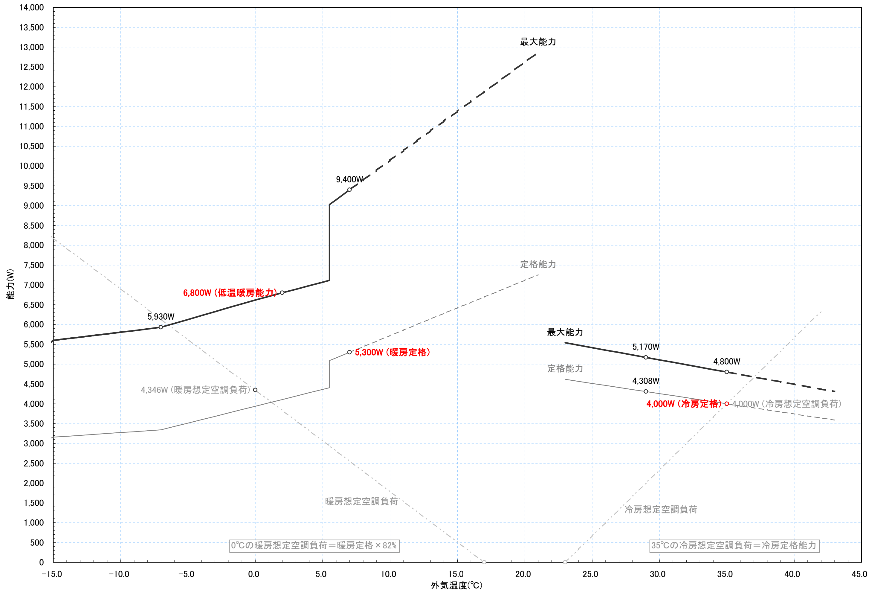
RAF-40Z2 冷暖房能力特性図 [室温 冷房:27°C一定, 暖房:20°C一定]
