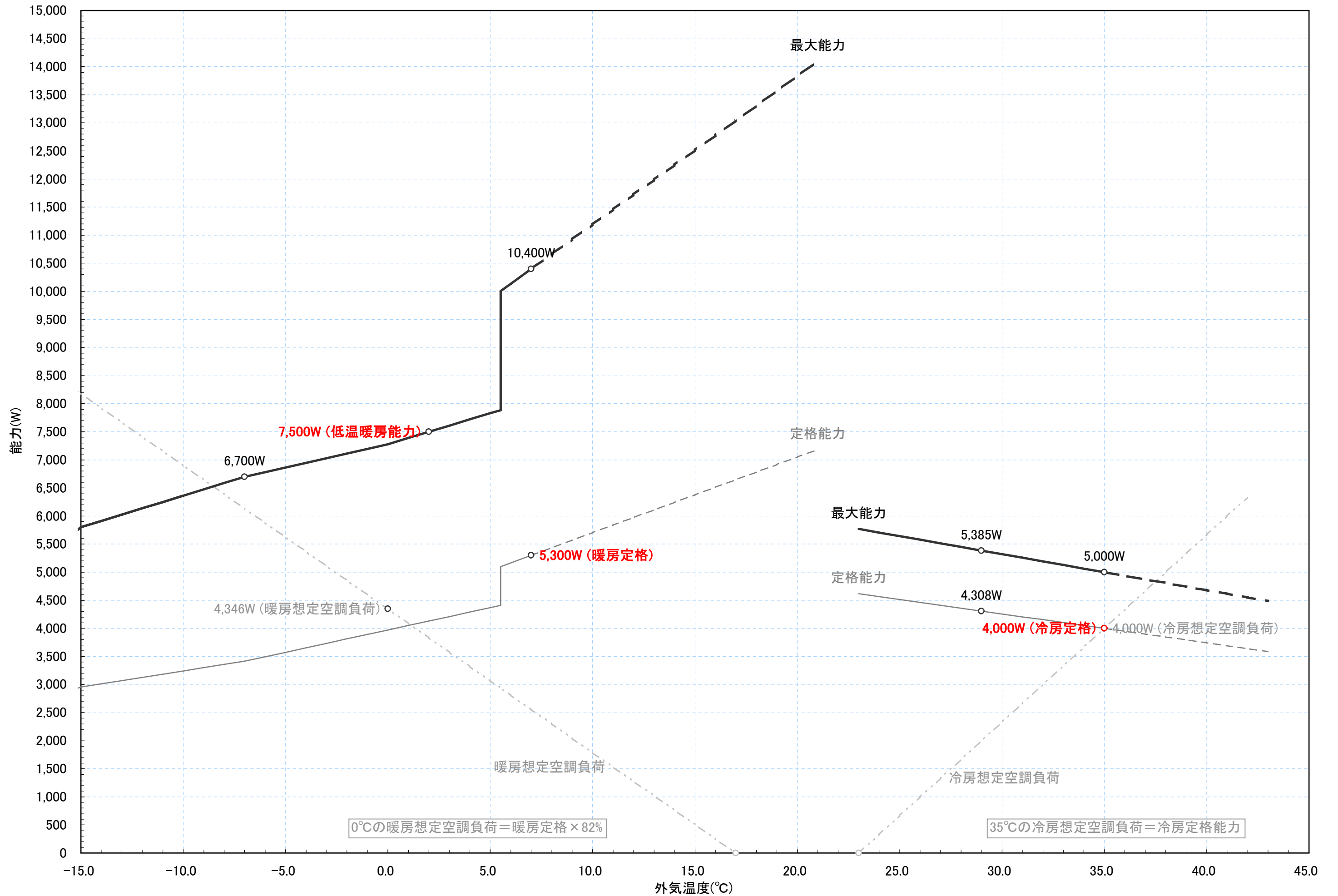
RAS-SD40Y2 冷暖房能力特性図 [室温 冷房:27°C一定, 暖房:20°C一定]
