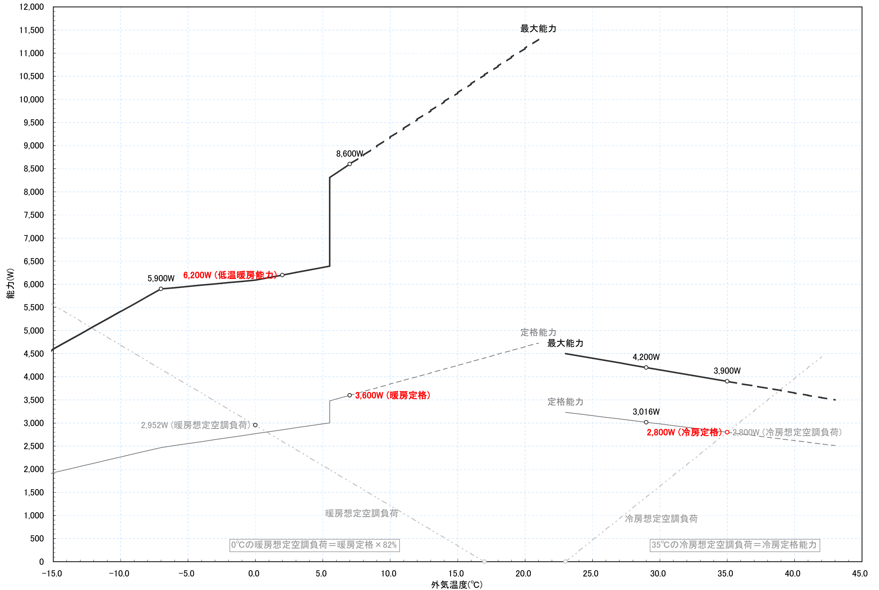
RAS-SD28Y2 冷暖房能力特性図 [室温 冷房:27°C一定, 暖房:20°C一定]
