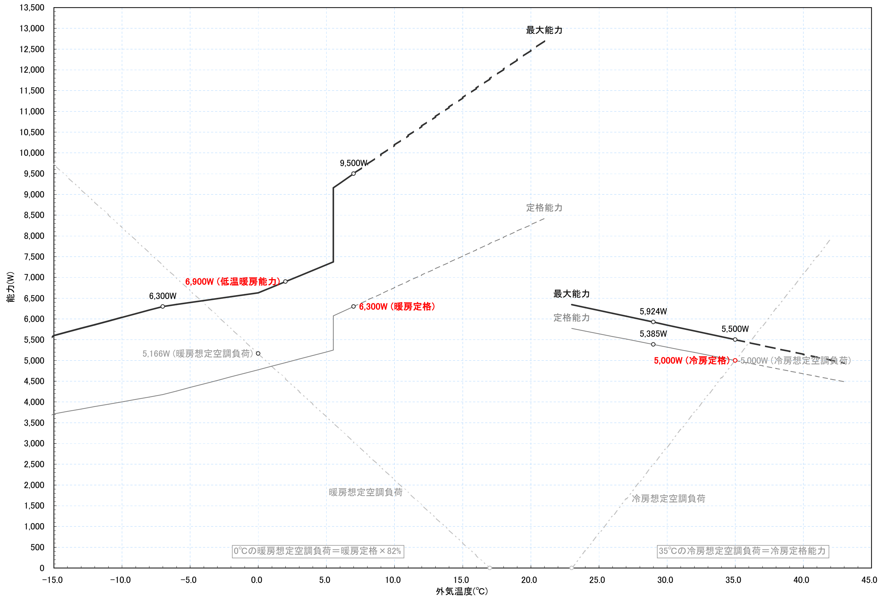
RAF-50Y2 冷暖房能力特性図 [室温 冷房:27°C一定, 暖房:20°C一定]
