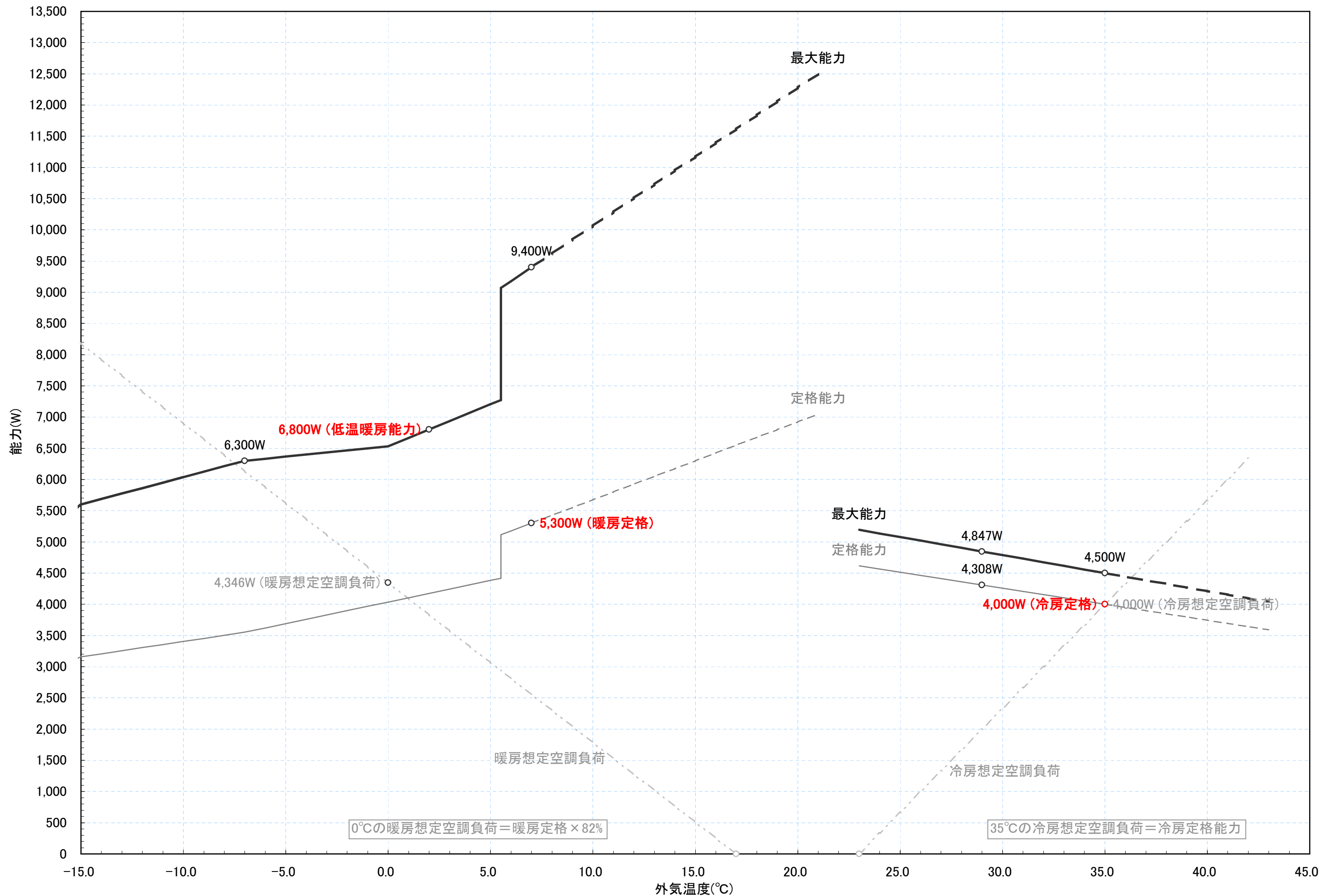
RAF-40Y2 冷暖房能力特性図 [室温 冷房:27°C一定, 暖房:20°C一定]
