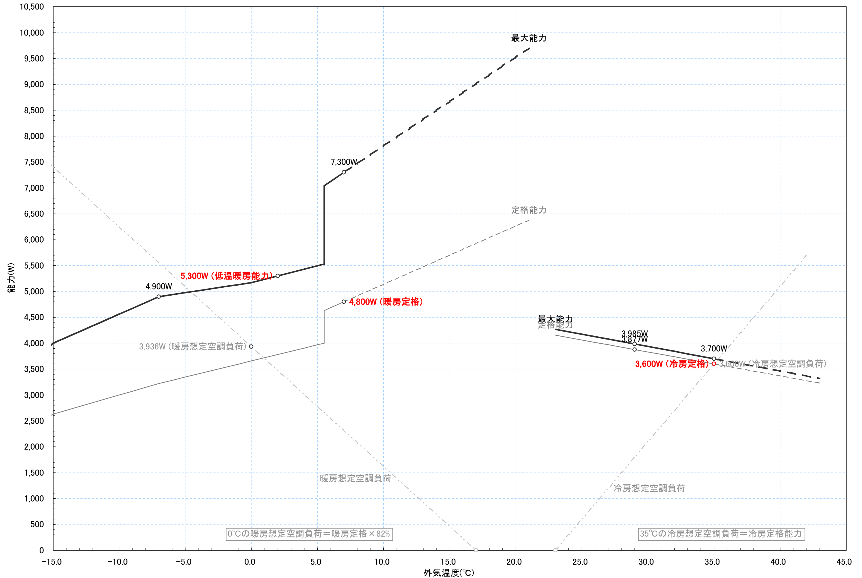
RAF-36Y 冷暖房能力特性図 [室温:冷房:27°C一定, 暖房:20°C一定]
