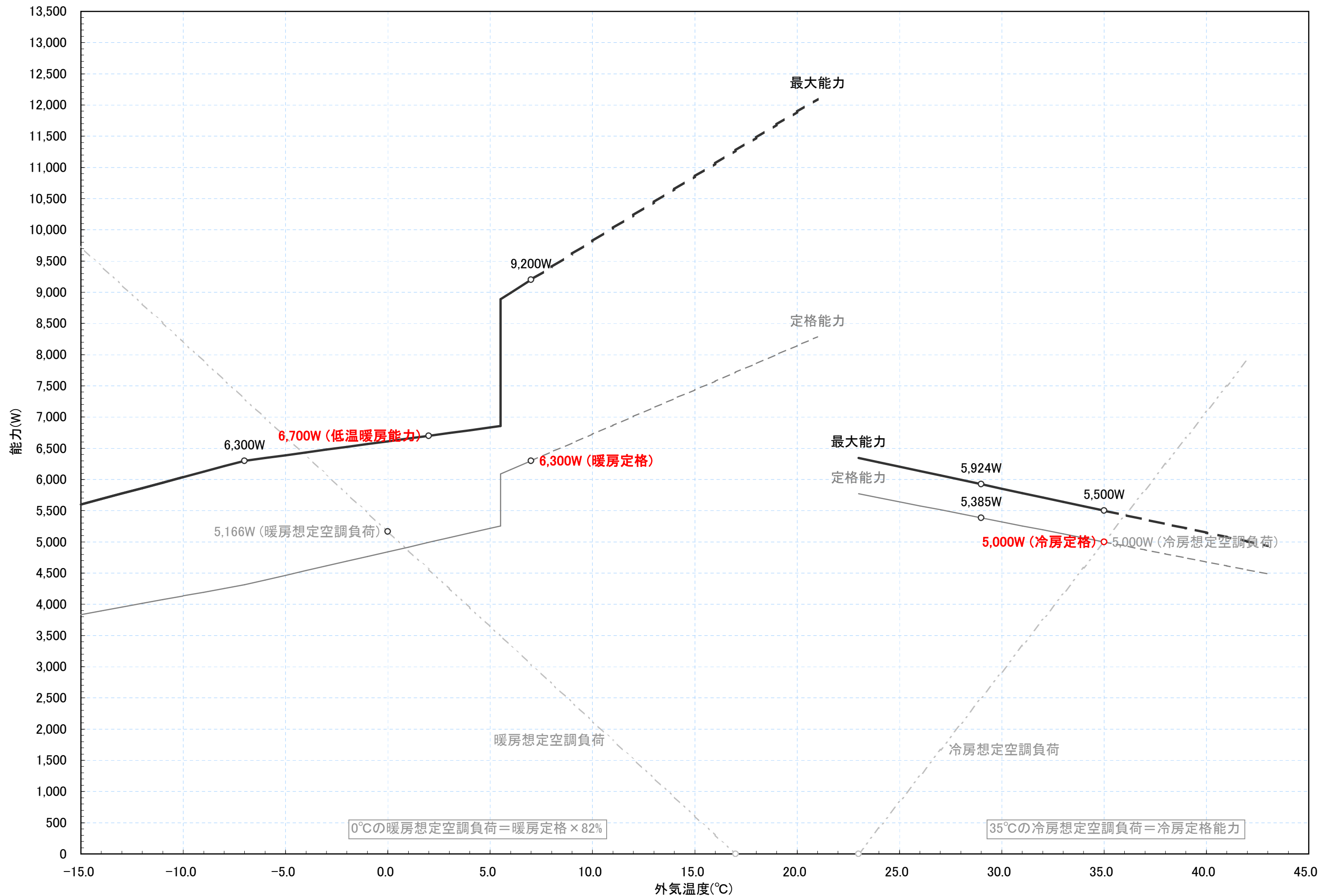
RAF-50X2 冷暖房能力特性図 [室温 冷房:27°C一定, 暖房:20°C一定]
