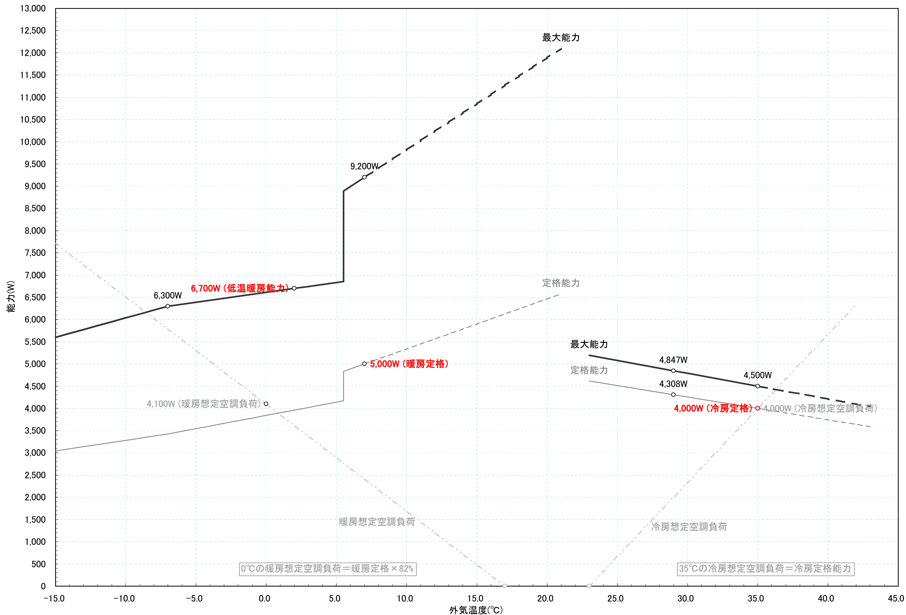
RAF-40X2 冷暖房能力特性図 [室温 冷房:27°C一定, 暖房:20°C一定]
