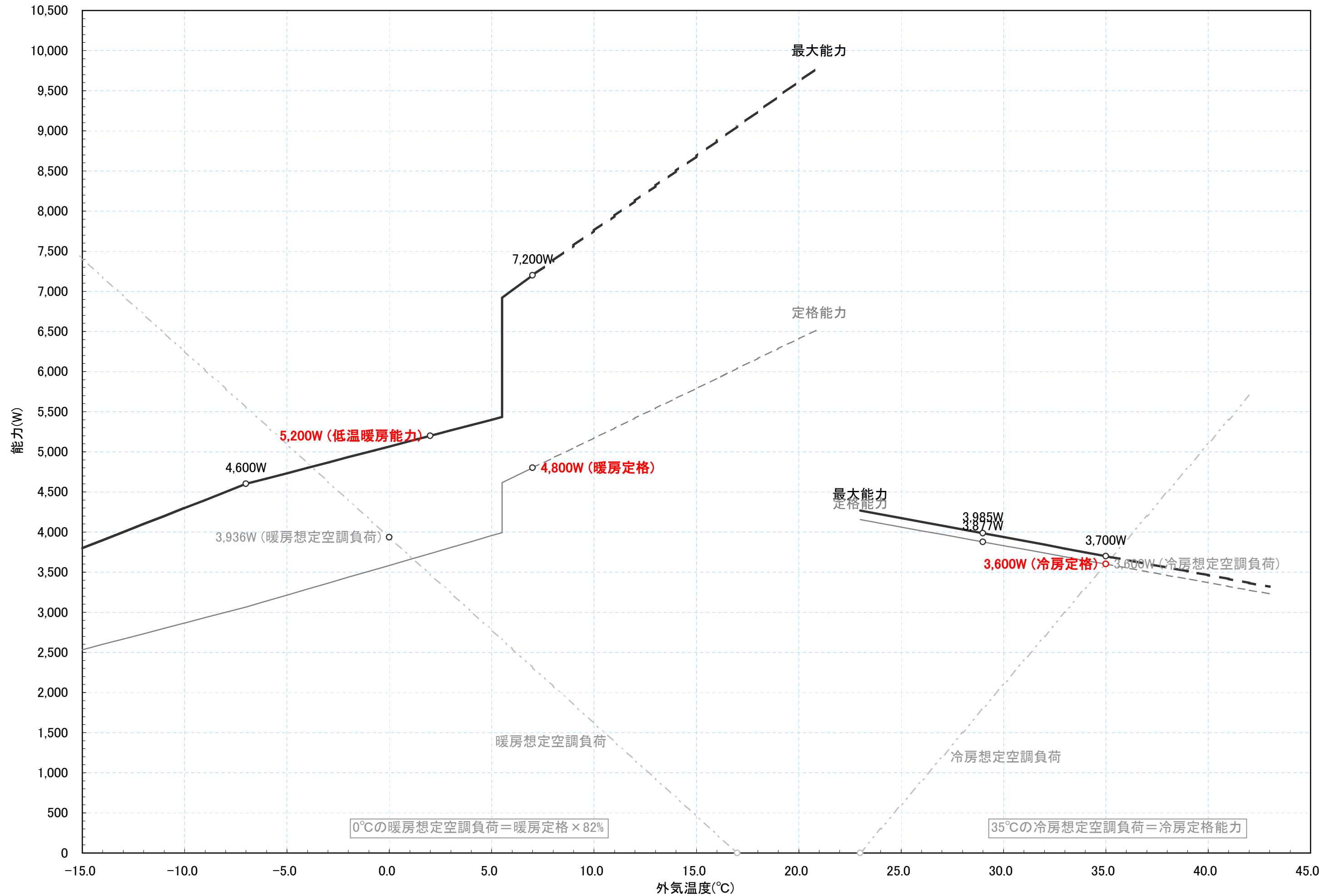
RAF-36X 冷暖房能力特性図 [室温:冷房:27°C一定, 暖房:20°C一定]
