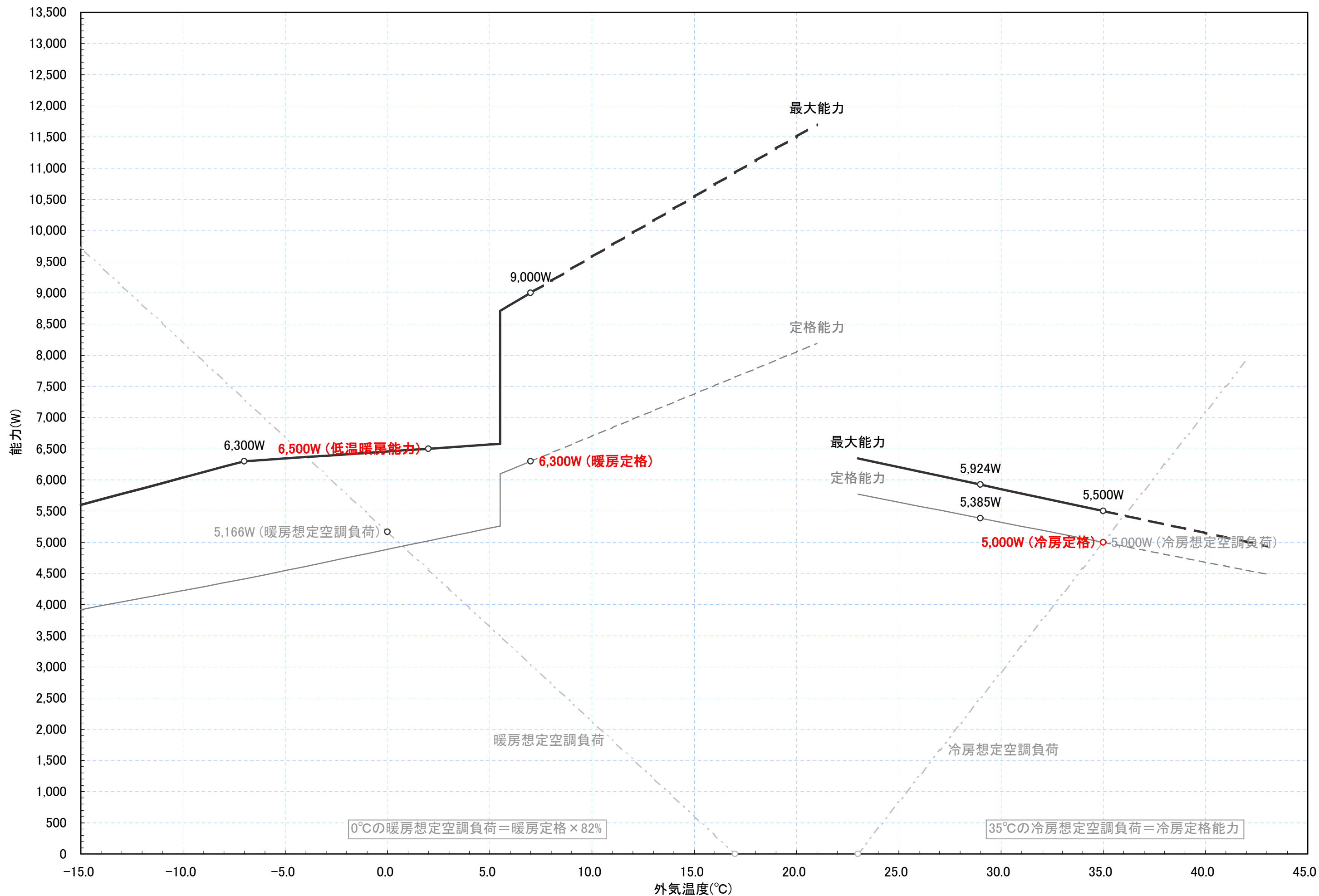
RAF-50W2 冷暖房能力特性図 [室温:冷房:27°C一定, 暖房:20°C一定]
