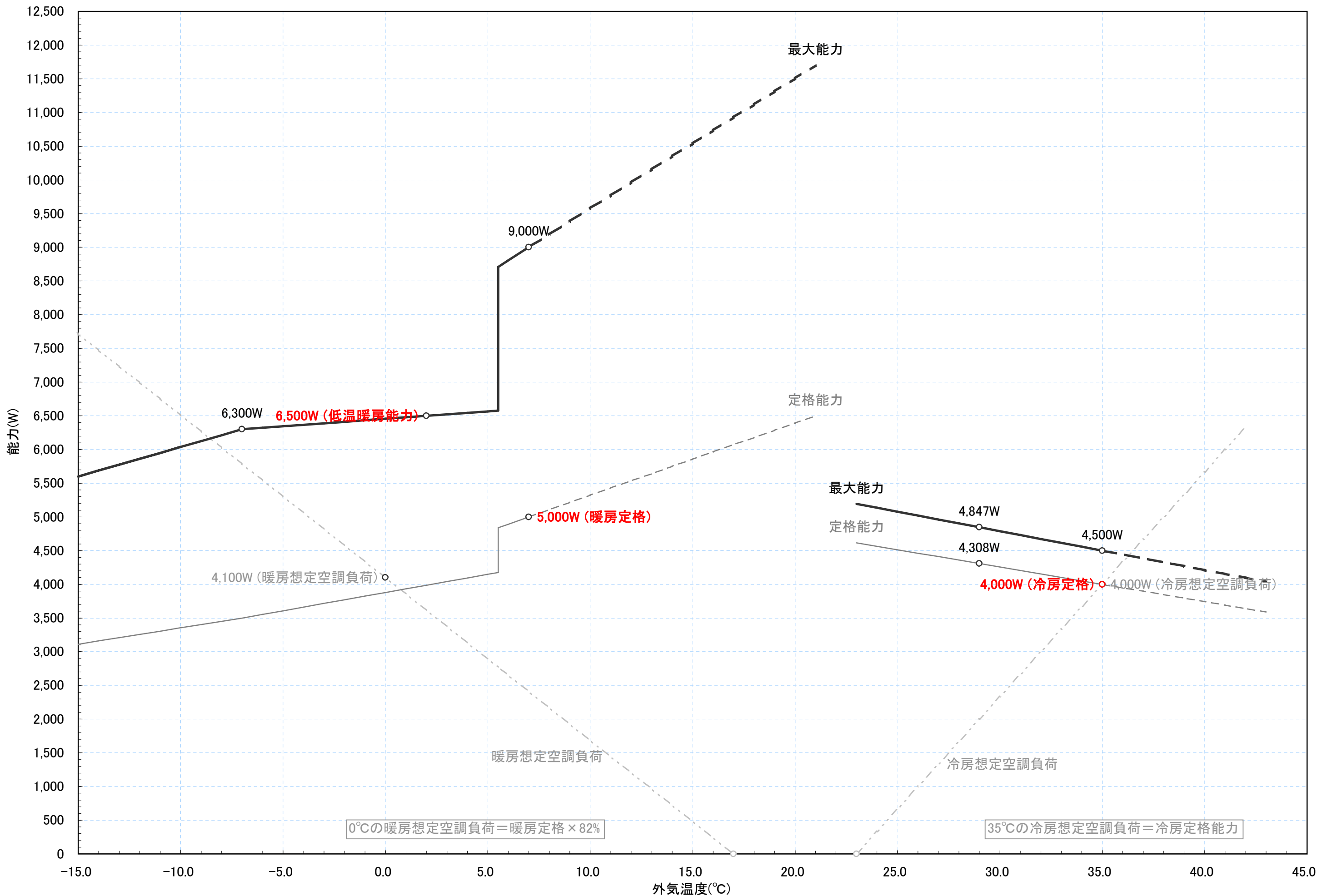
RAF-40W2 冷暖房能力特性図 [室温:冷房:27°C一定, 暖房:20°C一定]
